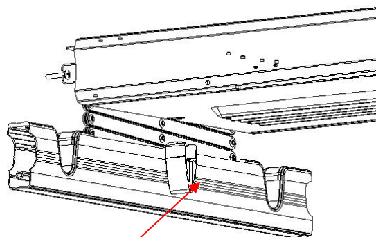
中间杆封口 图 11
